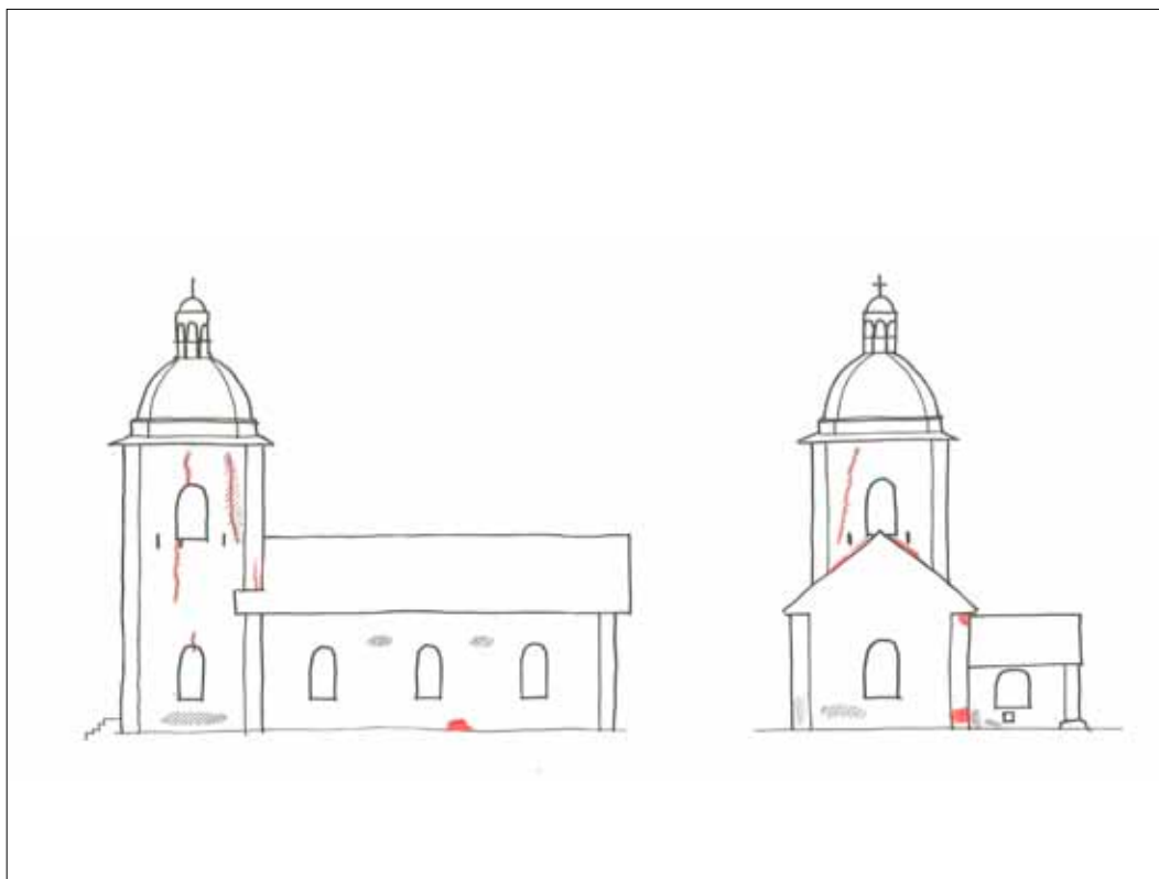
15 Skiss av Vagnhärads kyrkas södra och östra fasad. Röd markering är sprickor och putsskador och skrafferingar markerar entreprenörens lagningsdokumentation. Skiss Eva Wockatz.
