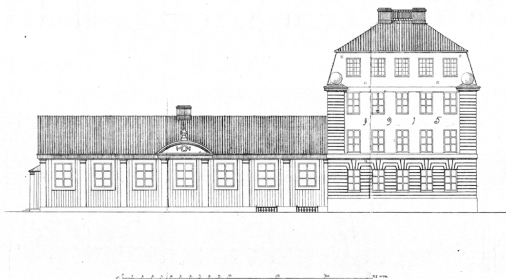
Ritning över D-skolans fasad mot nordost, godkänd av byggnadsnämnden 28 mars 1916. Gymnastikhuset, vilket var tänkt att byggas i trä, har en annan utformning än skolbyggnaden. Ritning från Oxelösunds kommun.
