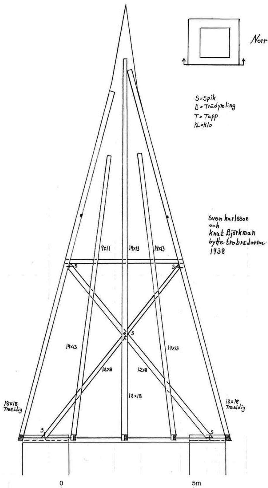
Uppmätning av timmerkonstruktionen sektion 2 vid tornhuvens östra sida från öster. Skalangivelsen till 1:50 i ritningshuvudet, gäller originalritningen. Bilden är förminskad, se därför skalstocken.
