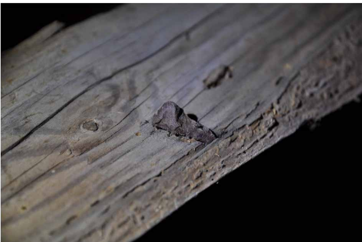
I södra högbenet på takstol 6 från öster, sitter en löst islagen spik, av samma typ som återfinns i Härad och Knista (Närke) kyrkor. Fotografi: Daniel Eriksson
