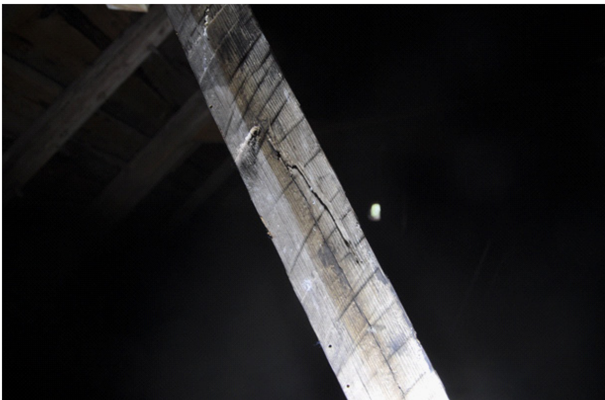
Stödben i form av halvklova. Man ser mårnen i mitten samt hornkvist. Fotografi: Daniel Eriksson
