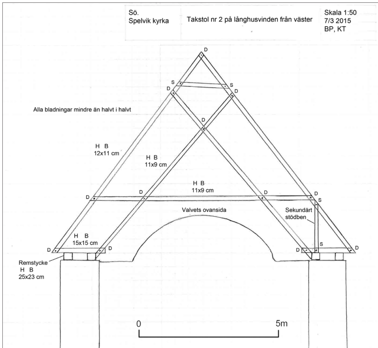
Uppmätning av takstol nummer 2 i långhuset. Skalangivelsen till 1:50 i ritningshuvudet, gäller originalritningen. Bilden är förminskad, se därför skalstocken.
