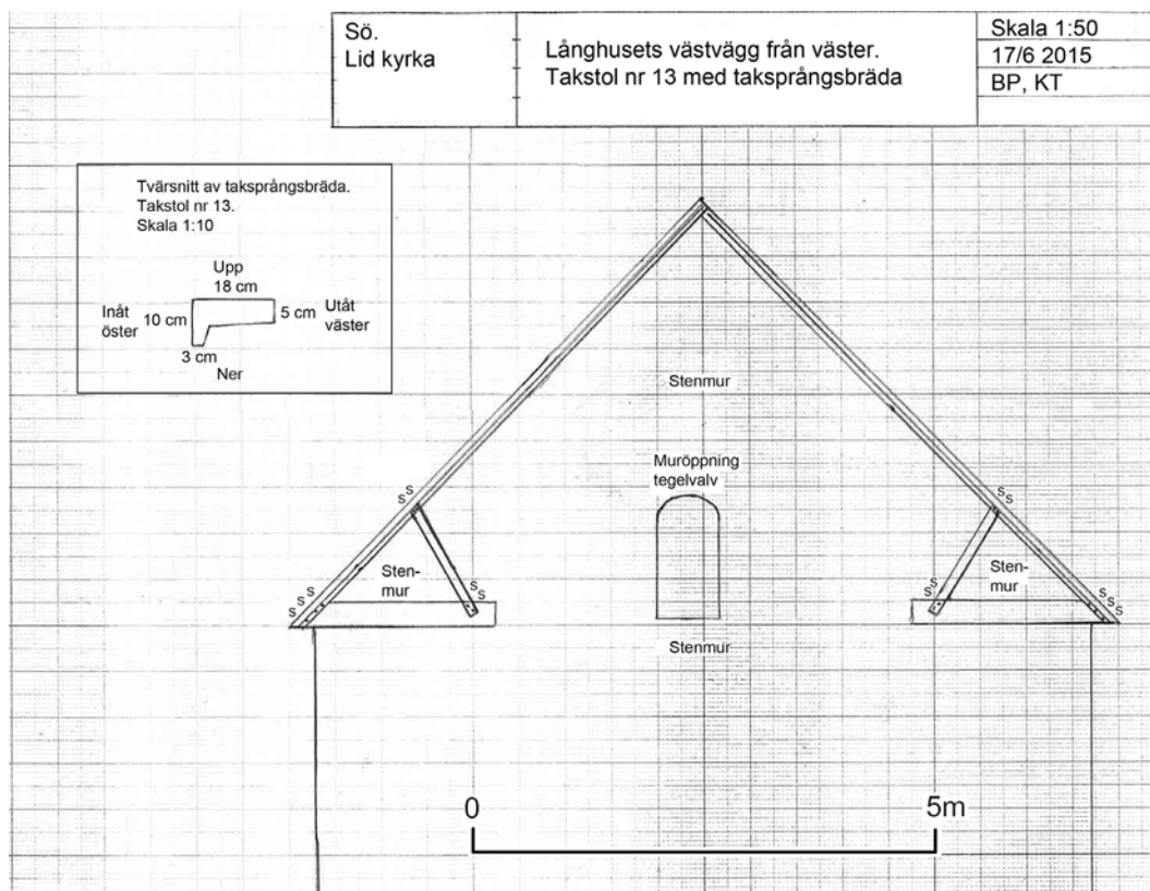
Uppmätning av takstol nr 13 i långhuset. Skalangivelserna till 1:50 i ritningshuvudet, gäller originalritningen. Bilden är förminskad, se därför skalstocken.
