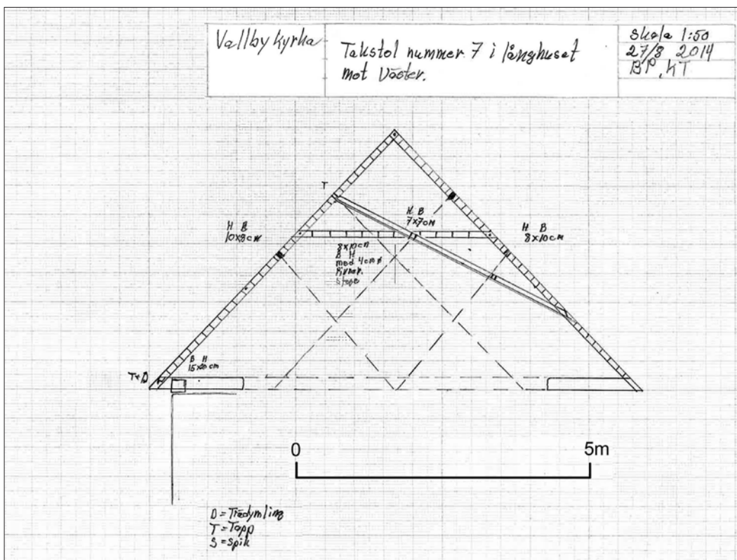
Uppmätning av takstol nummer 7 i den västra delen av långhuset. Skalangivelsen till 1:50 i ritningshuvudet, gäller originalritningen. Bilden är förminskad, se därför skalstocken.
