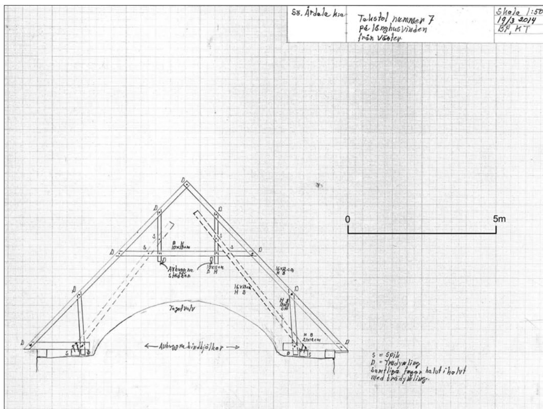
Uppmätning av taktol nummer 7 i långhuset, från väster. Skalangivelsen till 1:50 i ritningshuvudet, gäller originalritningen. Bilden är förminskad, se därför skalstocken.
