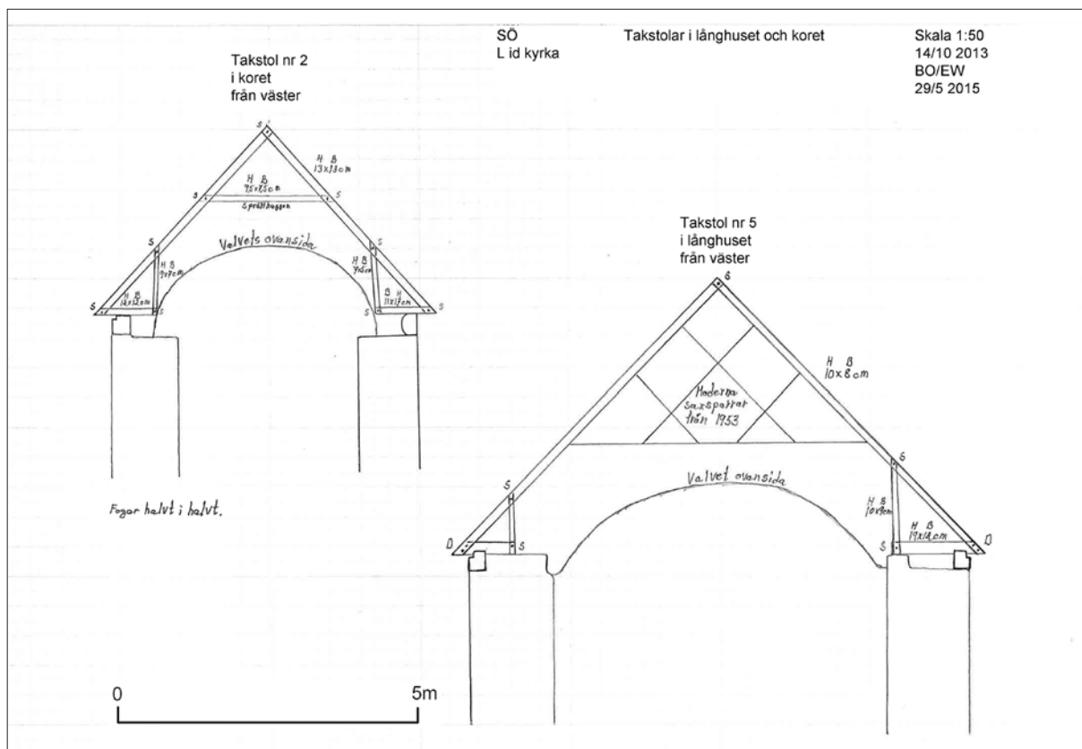
Uppmätning av takstol nr 5 i långhuset och takstol nr 2 koret. Skalangivelserna till 1:50 i ritningshuvudet, gäller originalritningen. Bilden är förminskad, se därför skalstocken.
