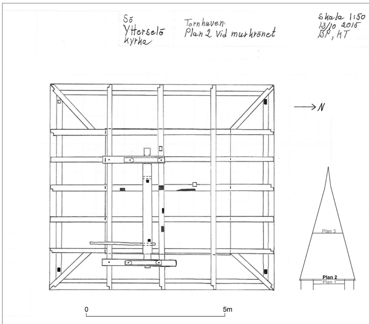
Uppmätning av tornhuvens timmerkonstruktion och klockvinsch i plan 2 vid murkrönet. Skalangivelsen till 1:50 i ritningshuvudet, gäller originalritningen. Bilden är förminskad, se därför skalstocken.
