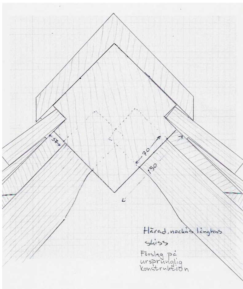
Rekonstruktion av den aktuella nockåsen i genomskärning med högbenen/sparrarna, taktro. På taktron ligger sedan spåntäckningen som går in i nockåsens fals. Överst en nockhuv.
