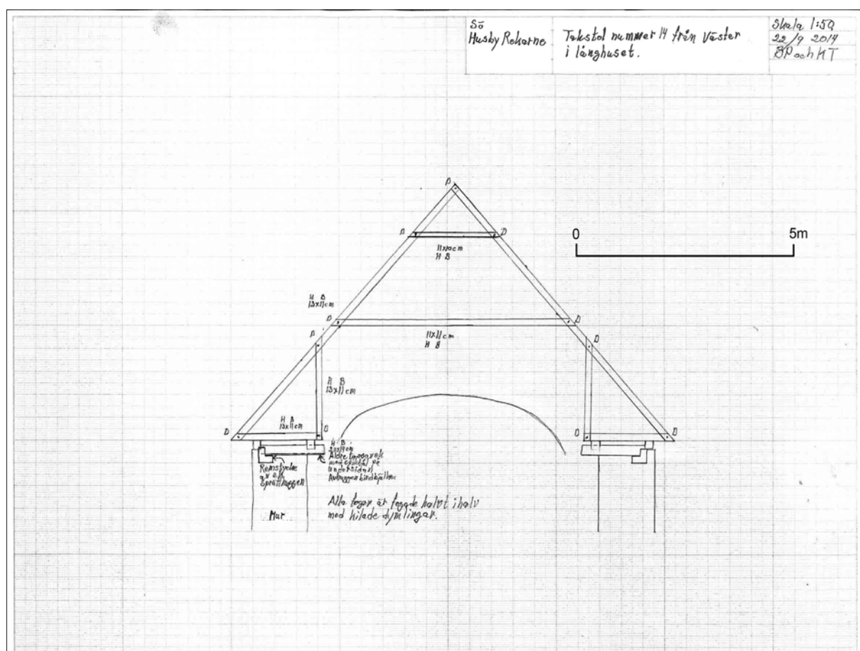
Uppmätning av takstol nummer 14 i långhuset från väster. Skalangivelsen till 1:50 i ritningshuvudet, gäller originalritningen. Bilden är förminskad, se därför skalstocken.
