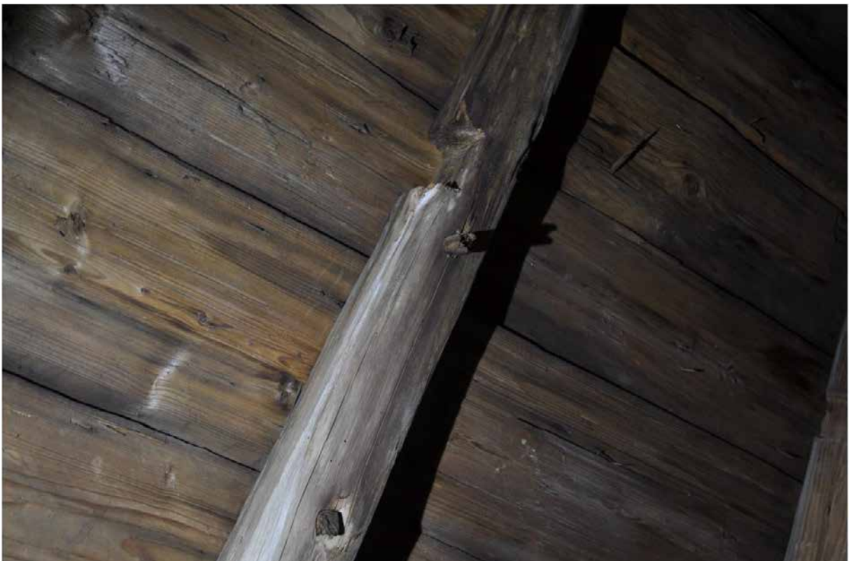
Även stödbenens infästning i högbenen har varit genomgående bladning med spik. Dymplingar för taktro finns fortfarande kvar. Ämnet till detta högben har troligen ej hållt måttet. Därför är undersidan helt obearbetad närmastnocken. Ganska ovanligt i romanska taklag. Fotografi: Daniel Eriksson
