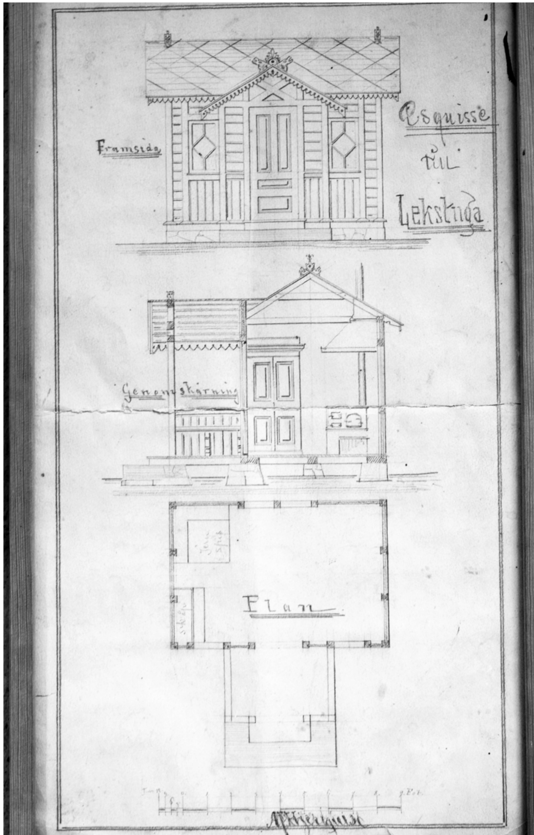
3 "Esquisse" av lekstugan. Ritningen är odaterad och ritad av AF Hjertquist. Ritning finns hos fastighetsägarna.
