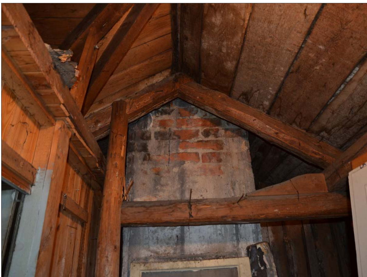
42 Vy upp i vindstaket sett mot norr. På den vänstra stolpen är det skrivet "1895". Till vänster är den tillbyggda delen med trapphus. Ovanpå underlagstaket syns näver, vilket kan anas till höger i bild (Slm D2014-306).
