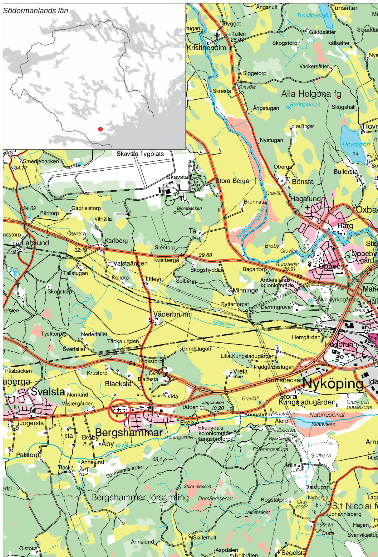
1 Utdrag ur Gröna kartans blad (GSD) Nyköping 9H SV med Bergshammars kyrka markerad. Skala 1:50 000.
