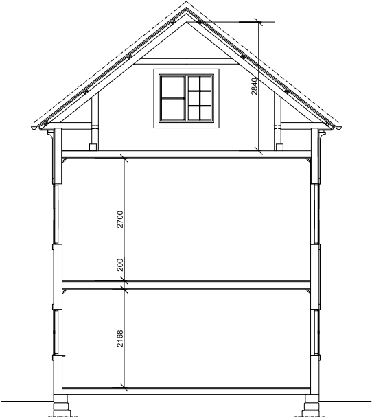
SEKTION A-A
