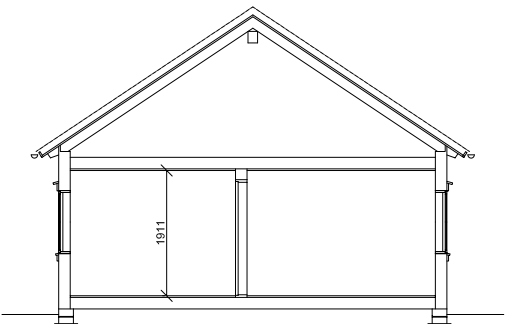
SEKTION A-A
