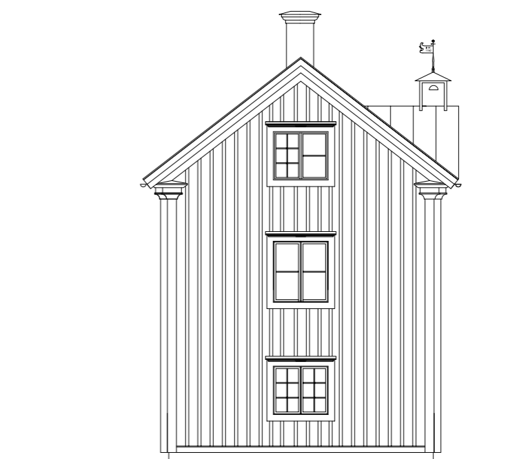
GAVEL MOT SÖDER
