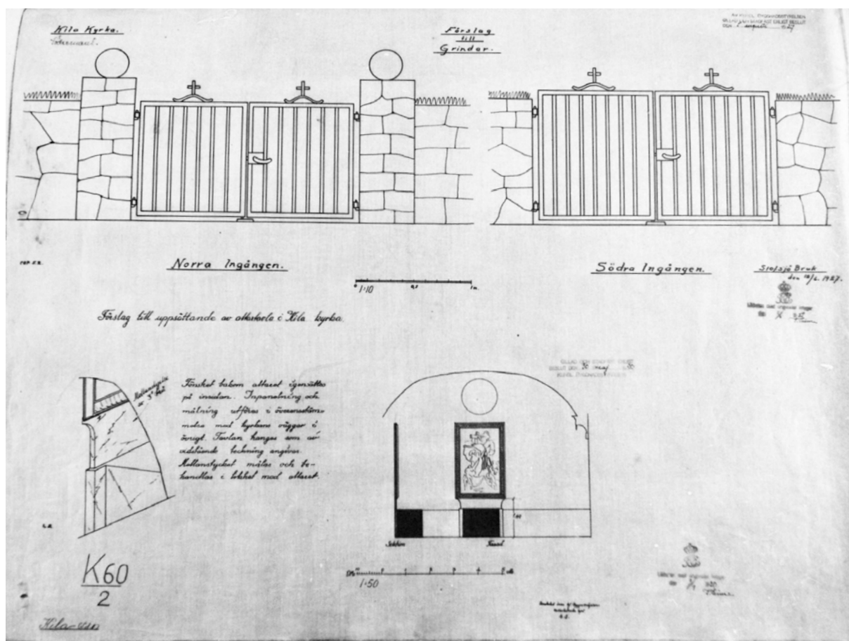
25 Ritningar på grindar av Aktiebolage Stafsjö Järnväg, vilka även tillverkade grindarna. RAÄ, ATA. Ritning K 60.2.
